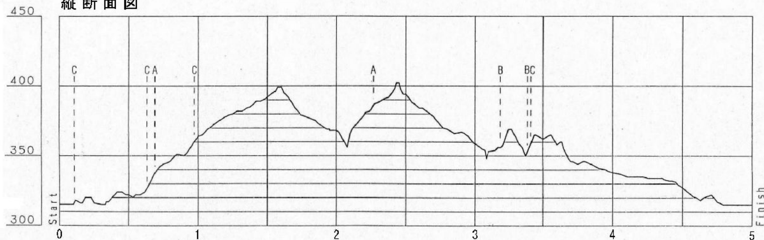
縦断面図
