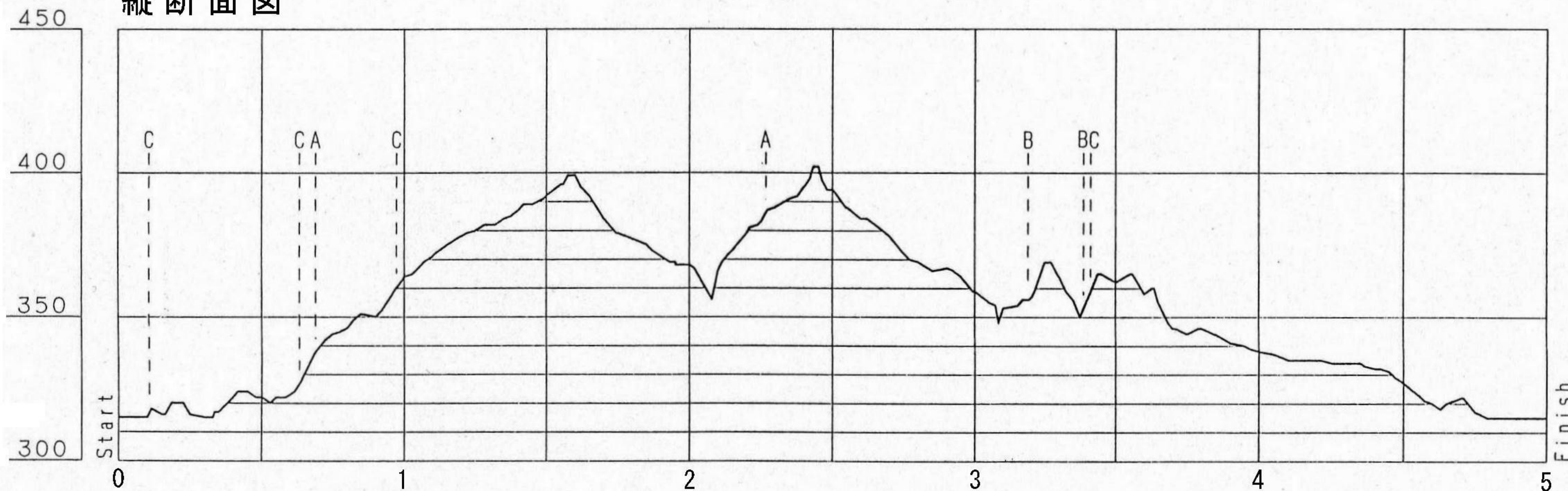
縦断面図
