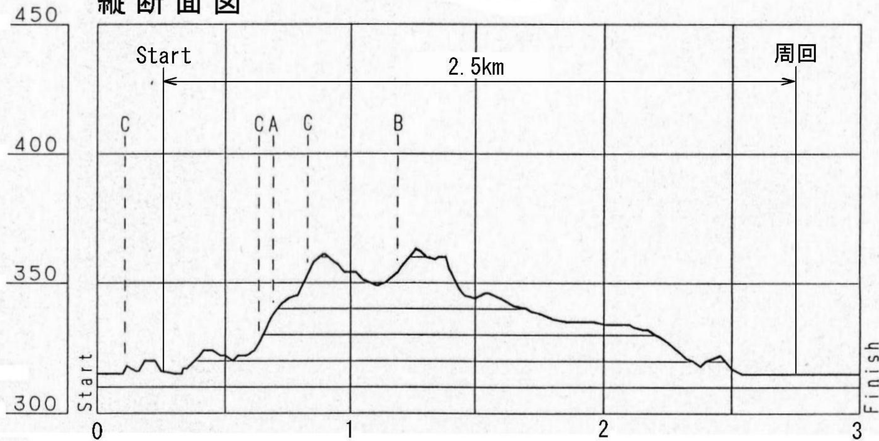
縦断面図
